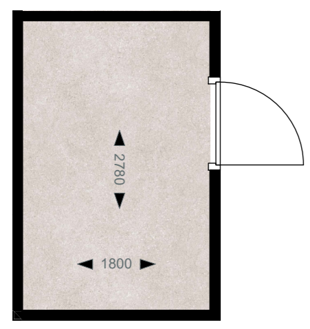
berging - schaal 1:50
